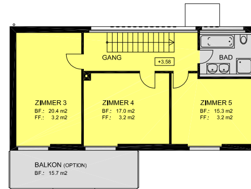
Obergeschoss
