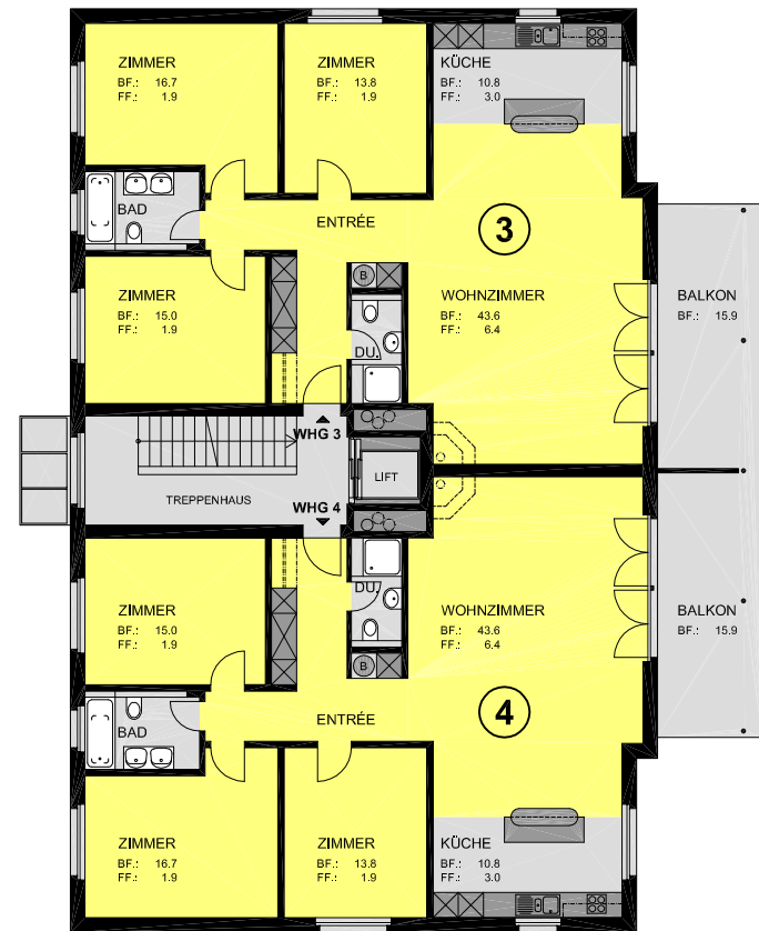
1. Obergeschoss
