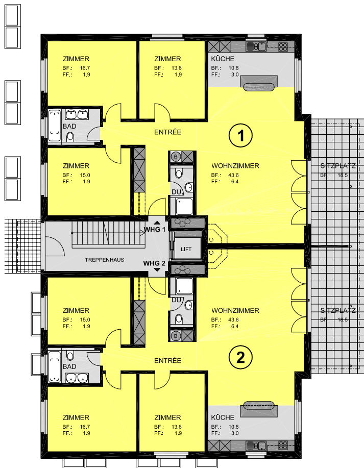
Erdgeschoss
