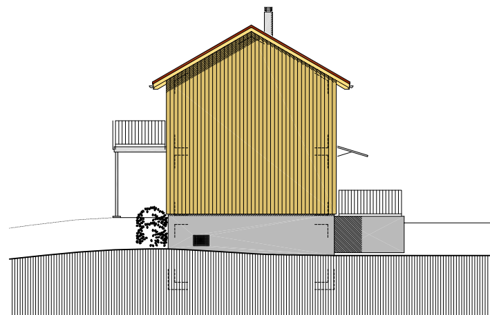
Ostfassade
