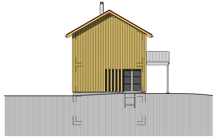
Westfassade
