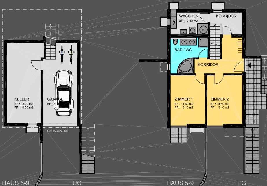
Grundrisse 1:200 Grosse, helle Zimmer. Viel platzbietendes Bade- zimmer mit Eckbadewanne. Geräumige Keller.
