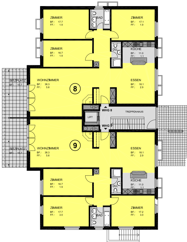
Erdgeschoss
