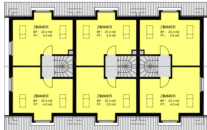
Dachgeschoss
