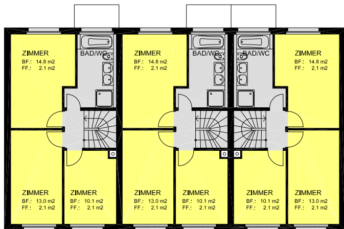
Obergeschoss
