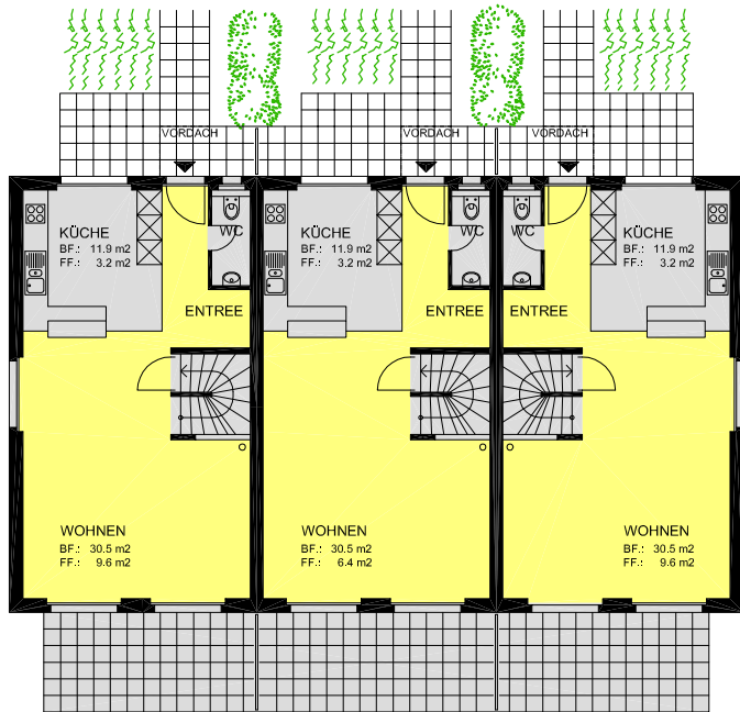
Erdgeschoss
