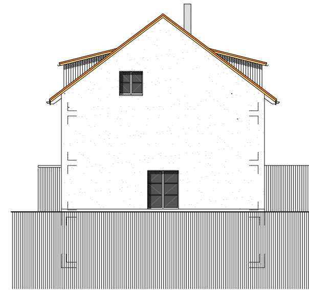
Südfassade
