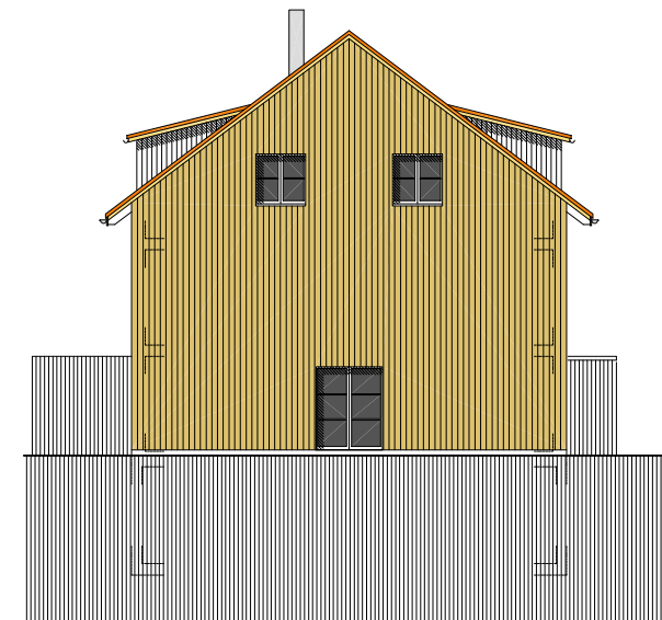
Nordfassade
