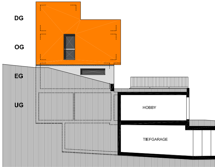
Westfassade
