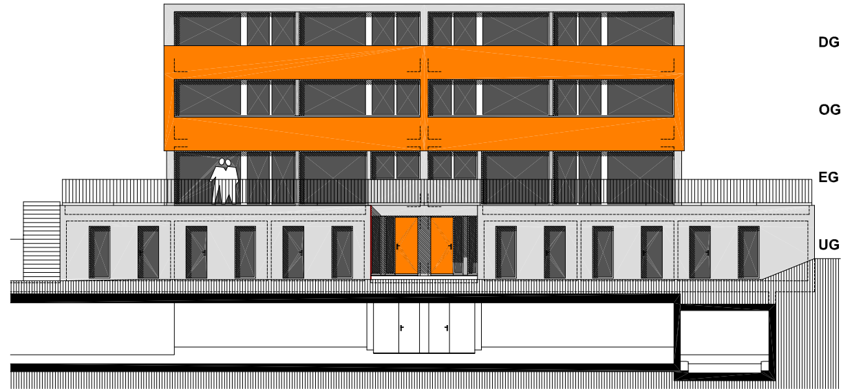
Südfassade
