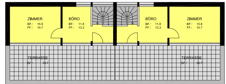
Dachgeschoss
