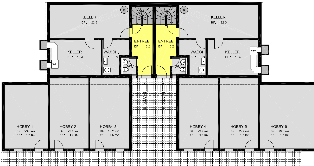
Untergeschoss
