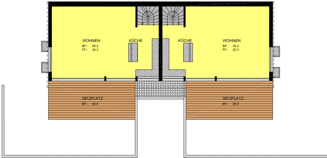
Erdgeschoss
