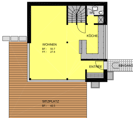
Erdgeschoss
